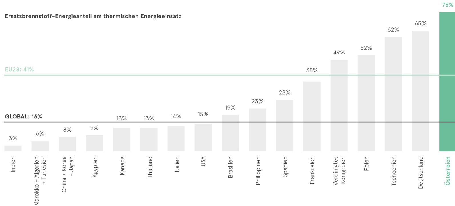
ERSATZBRENNSTOFFRATE DER ZEMENTINDUSTRIE IM INTERNATIONALEN VERGLEICH (2014)
